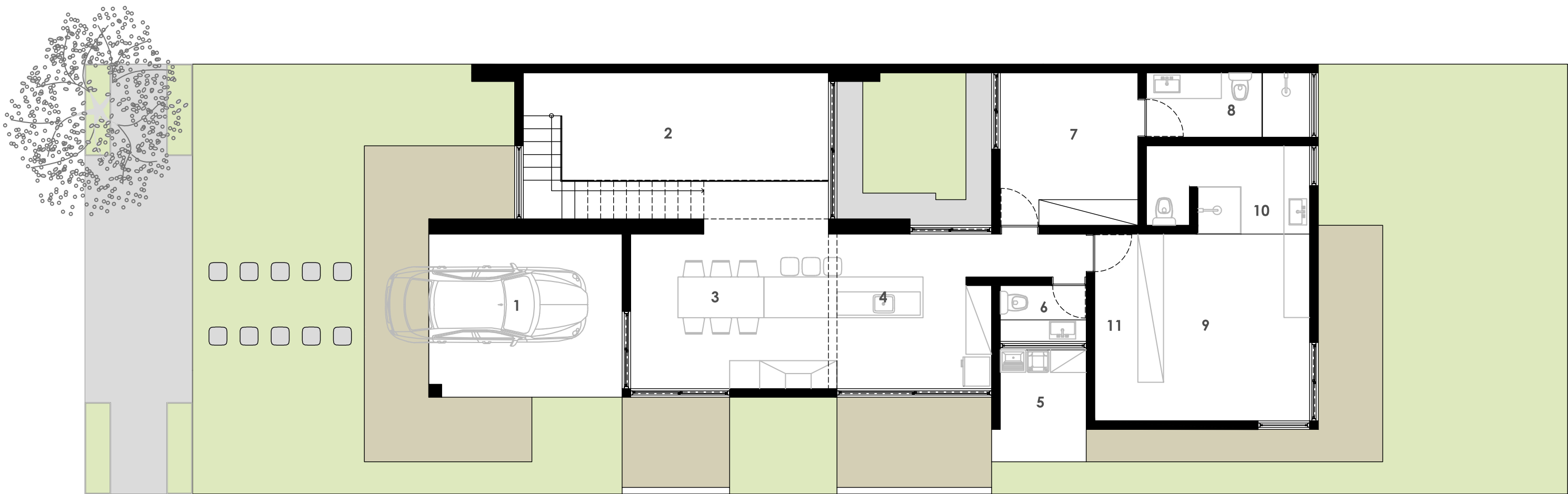
Planta térreo Sem escala
